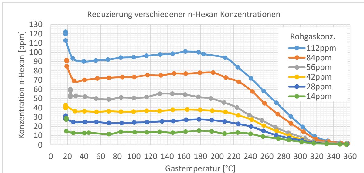
Abbildung 15: Ergebnisse der Versuche zur n -Hexan-Reduktion mittels katalytischem Verfahren, Änderung der n -Hexankonzentration in Abhängigkeit der Gastemperatur
