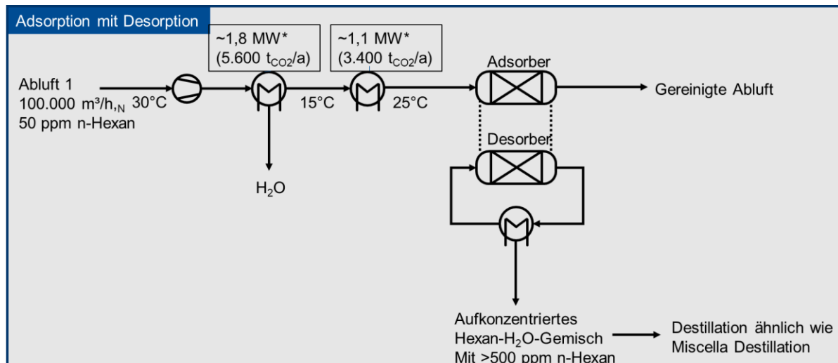
Abbildung 26: Möglicher Prozesspfad: Adsorption mit Desorption. * Ideal (Ohne Wirkungsgrade und Abwärmeverluste, CO 2 -Faktor deutscher Strommix: 353 g/kWh)
