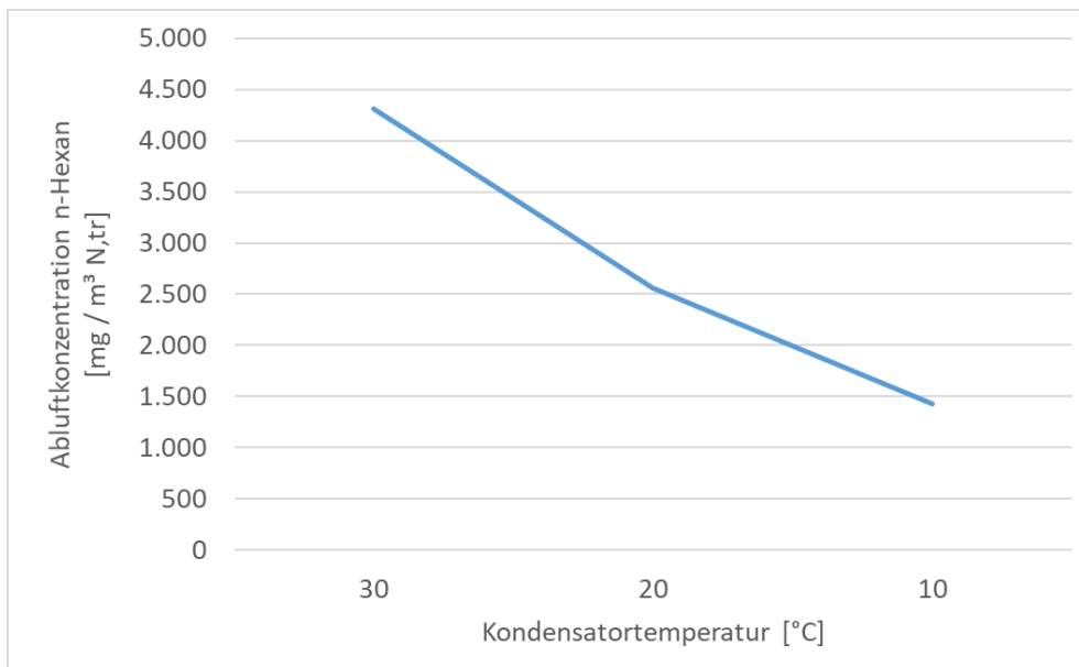
Abbildung 25: Berechnete n -Hexankonzentration in Abluft 2 in Abhängigkeit der Kondensatortemperatur
