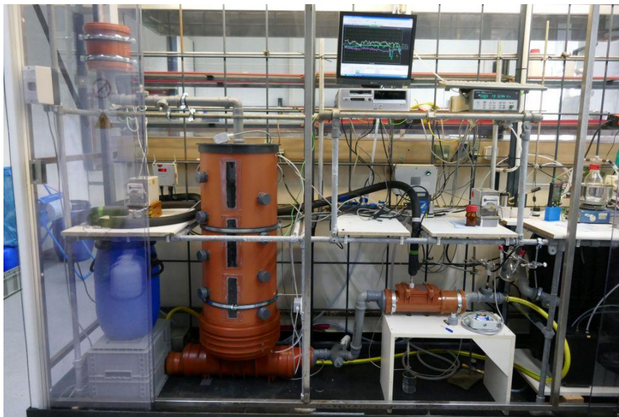
Abbildung 5: Biofilterlaboranlage – Skizze und Foto
