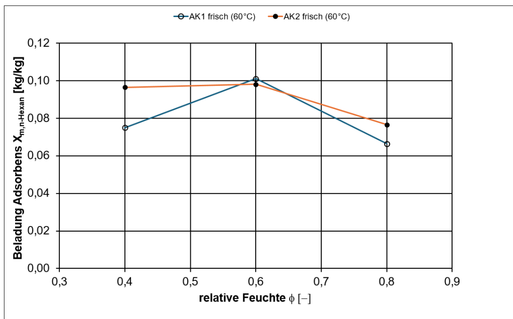
Abbildung 11: Gleichgewichtsbeladung bei variierender relativer Feuchte, Temperatur: 60°C, Konzentration: 42 ppm n -Hexan (150 mg/Nm 3 ), Volumenstrom: 5l/min
