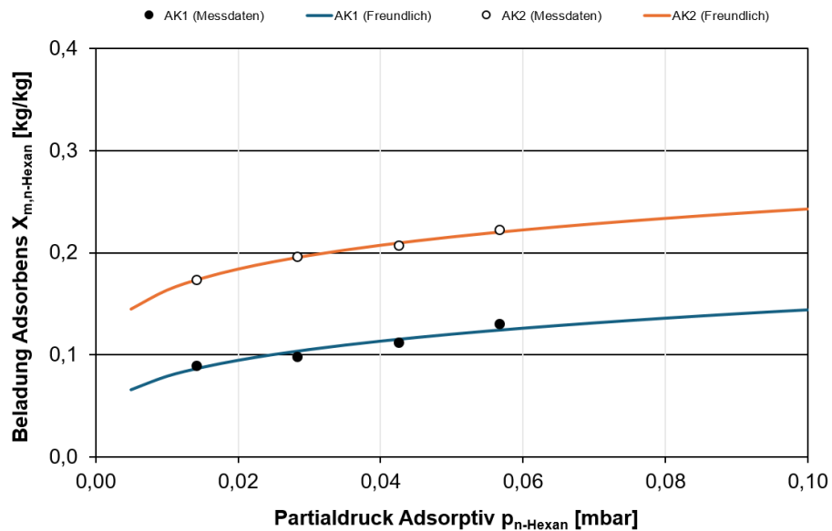
Abbildung 9: Freundlich-Adsorptionsisothermen für AK1 (Jacobi) und AK2 (Adsor-Tech) bei 25°C, Feuchte: 40%, Volumenstrom: 5 l/min
