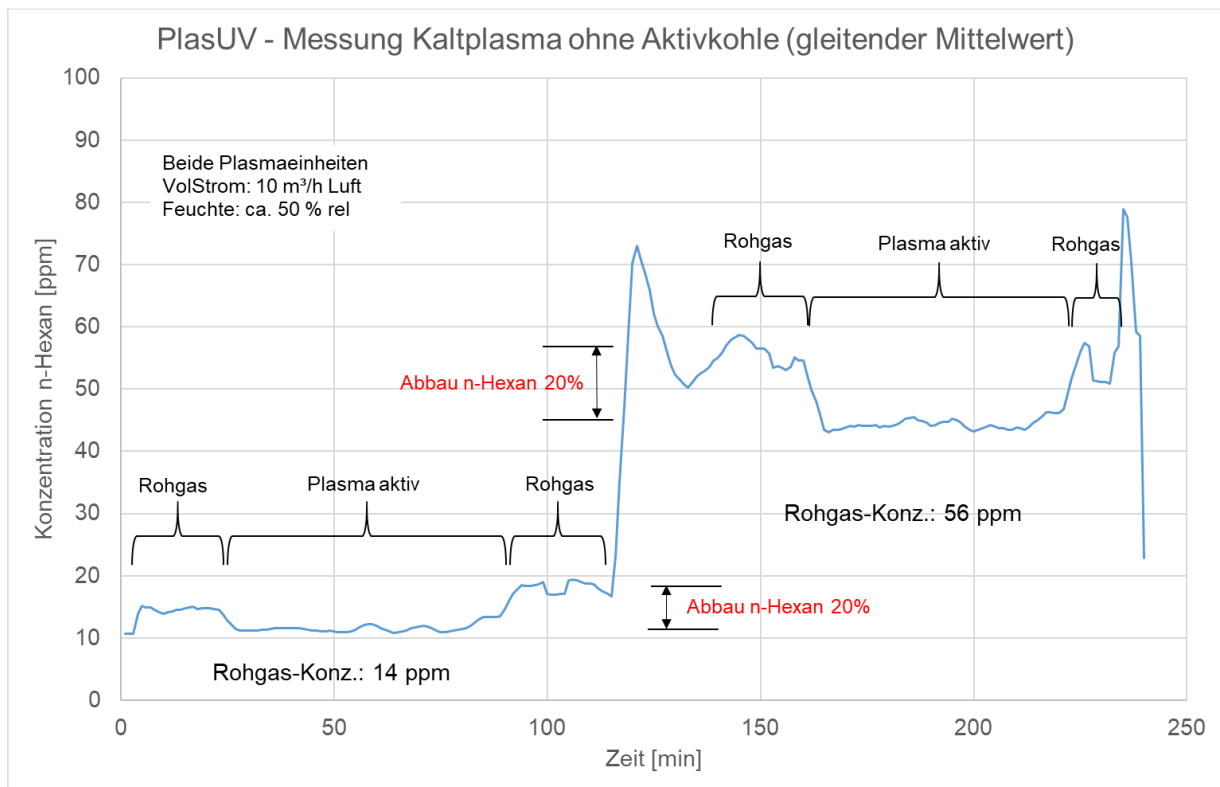
Abbildung 4: Verlauf der n -Hexan-Konzentration am Ausgang der Kaltplasmaversuchsanlage ohne Aktivkohle bei 14 und 56 ppm n -Hexan, 20 °C, 50 % rF
