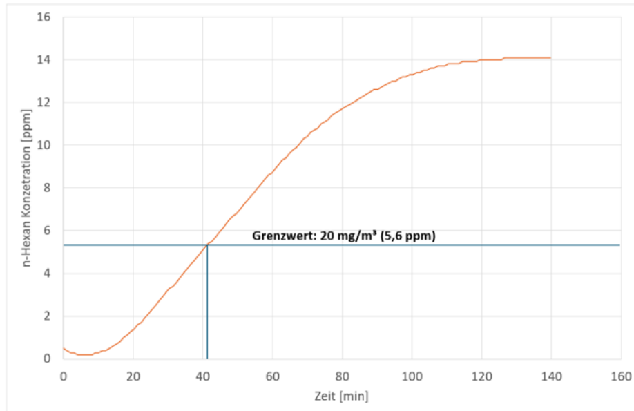
Abbildung 8: Durchbruchskurve AK2 (Adsor-Tech Aktivkohle) mit Beaufschlagung von 14 ppm n -Hexan (50 mg/m 3 ), m_{AK}=0,075\text{g} , V'=5\text{l/min} , Feuchte: 40% errechnete Gleichgewichtsbeladung: 0,2 g n -Hexan /g AK
