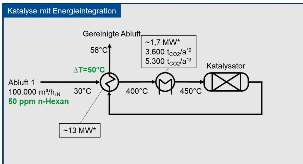
Abbildung 27: Möglicher Prozesspfad: Katalyse. * Ideal (Ohne Wirkungsgrade und Abwärmeverluste), ^{*2} Erdgas- \text{CO}_2 -Faktor: 242 \text{ g/kWh} , ^{*3} \text{CO}_2 -Faktor deutscher Strom-Mix: 353 \text{ g/kWh}
