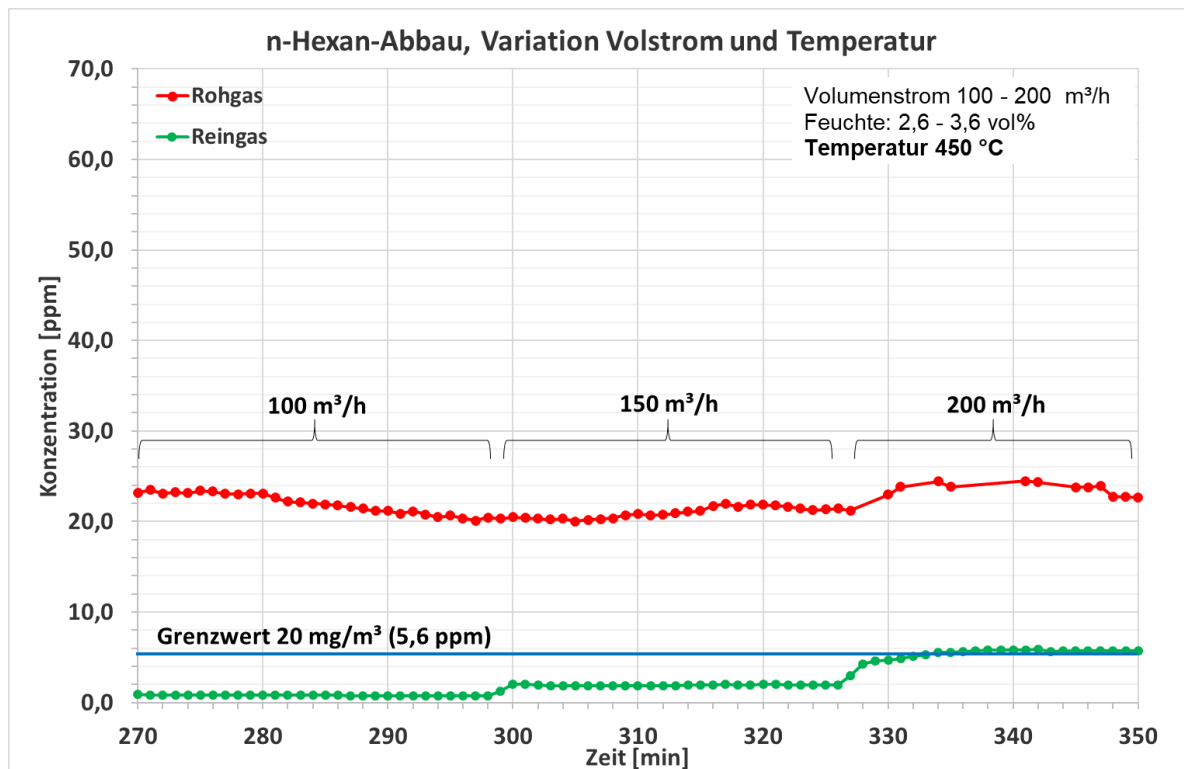
Abbildung 20: Realgasmessung, Temperatur 450°C, Volumenstrom 100, 150, 200 m³/h
