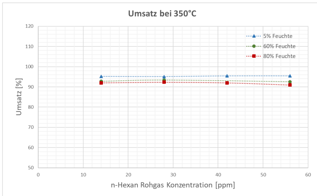
Abbildung 16: Ergebnisse der Versuche zur n -Hexan-Reduktion mittels katalytischem Verfahren, Darstellung des Einflusses der Feuchte auf den Umsatz bei einer Katalysatortemperatur von 350°C
