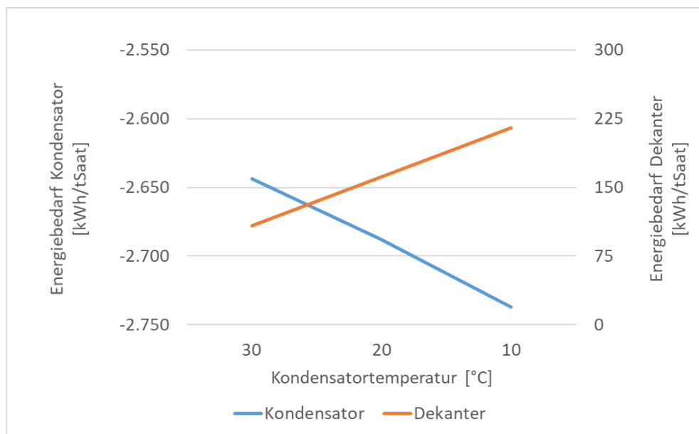
Abbildung 24: Berechneter Energiebedarf von Kondensator und Dekanter bei Variation der Kondensatortemperatur
