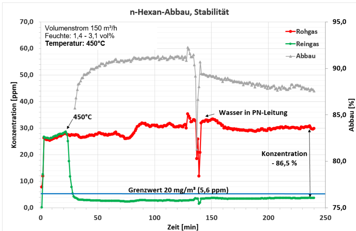
Abbildung 21: Realgasmessung, Temperatur 450°C, Volumenstrom 150 m³/h
