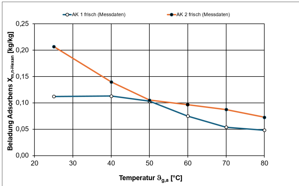
Abbildung 12: Gleichgewichtsbeladung bei variierender Temperatur zwischen 25-80°C, Konzentration: 42 ppm n -Hexan (150 mg/Nm 3 ), Volumenstrom: 5l/min, Feuchte: 40%
