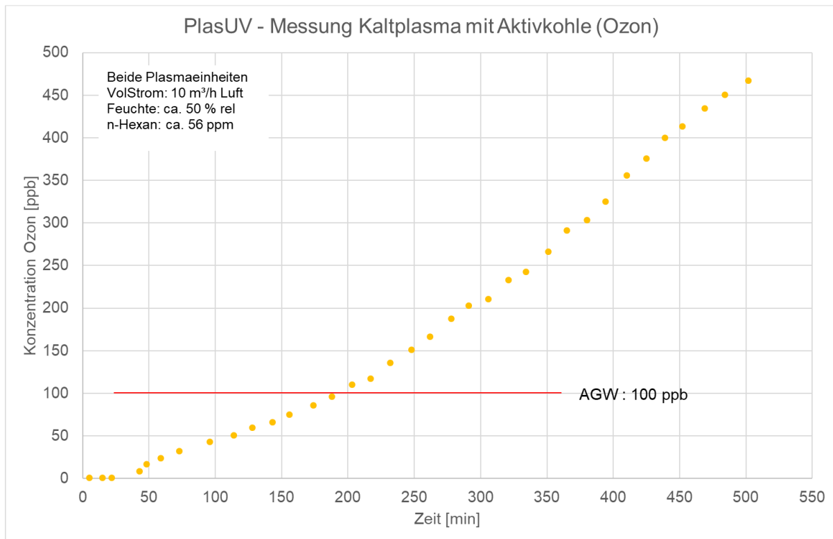
Abbildung 3: Verlauf der Ozonkonzentration am Ausgang der Kaltplasmaversuchsanlage bei ca. 56 ppm n -Hexan (200 mg/m³), 20 °C, 50 % rF
