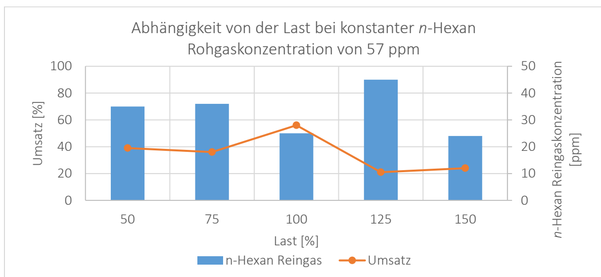
Abbildung 6: Ergebnisse der Biofilterversuche
