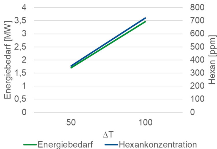
Abbildung 28: Energiebedarf in Abhängigkeit zum Temperaturgradienten des Vorwärmers sowie die dazu korrespondierende n -Hexan-Konzentration für einen autothermen Betrieb
