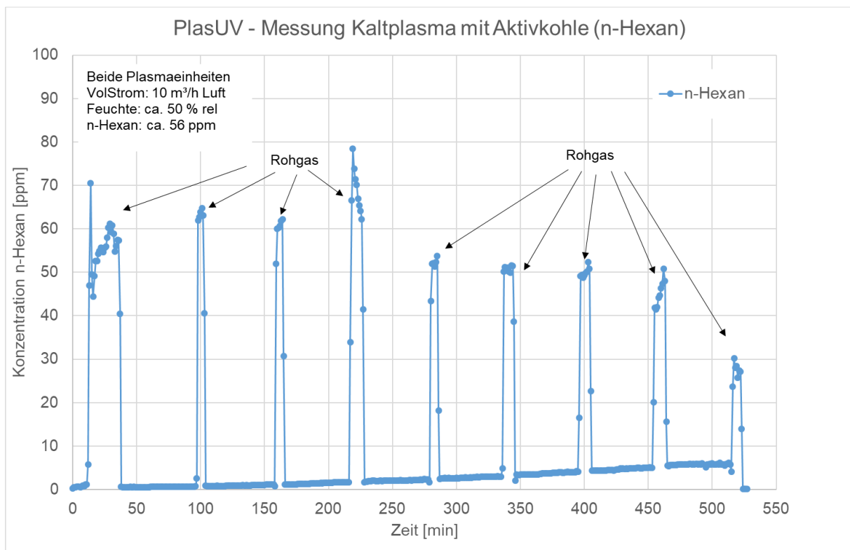
Abbildung 2: Verlauf der n -Hexan-Konzentration am Ausgang der Kaltplasmaversuchsanlage bei ca. 56 ppm n -Hexan (200 mg/m 3 ), 20 °C, 50 % rF
