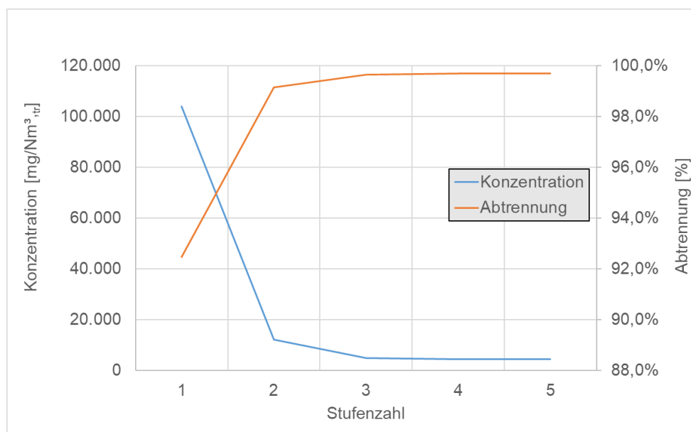
Abbildung 23: Absorption in Abhängigkeit der Stufenzahl
