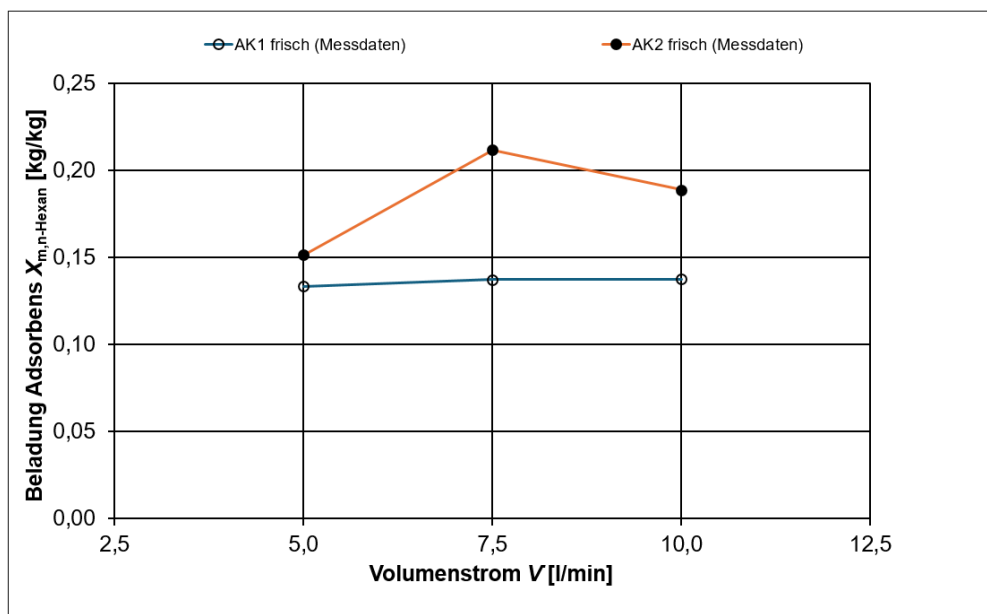
Abbildung 13: Gleichgewichtsbeladung bei variierendem Volumenstrom zwischen 5-10 l/min, Temperatur: 25°C, Konzentration: 42 ppm n -Hexan (150 mg/Nm 3 ), Feuchte: 40%
