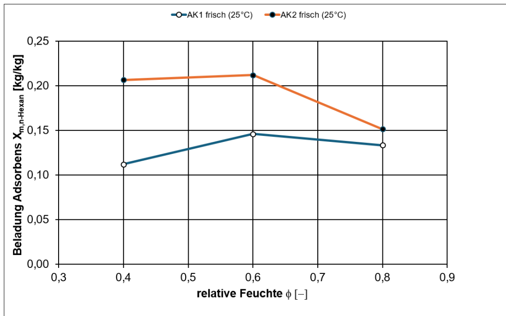
Abbildung 10: Gleichgewichtsbeladung bei variierender relativer Feuchte, Temperatur: 25°C, Konzentration: 42 ppm n -Hexan (150 mg/Nm 3 ), Volumenstrom: 5l/min
