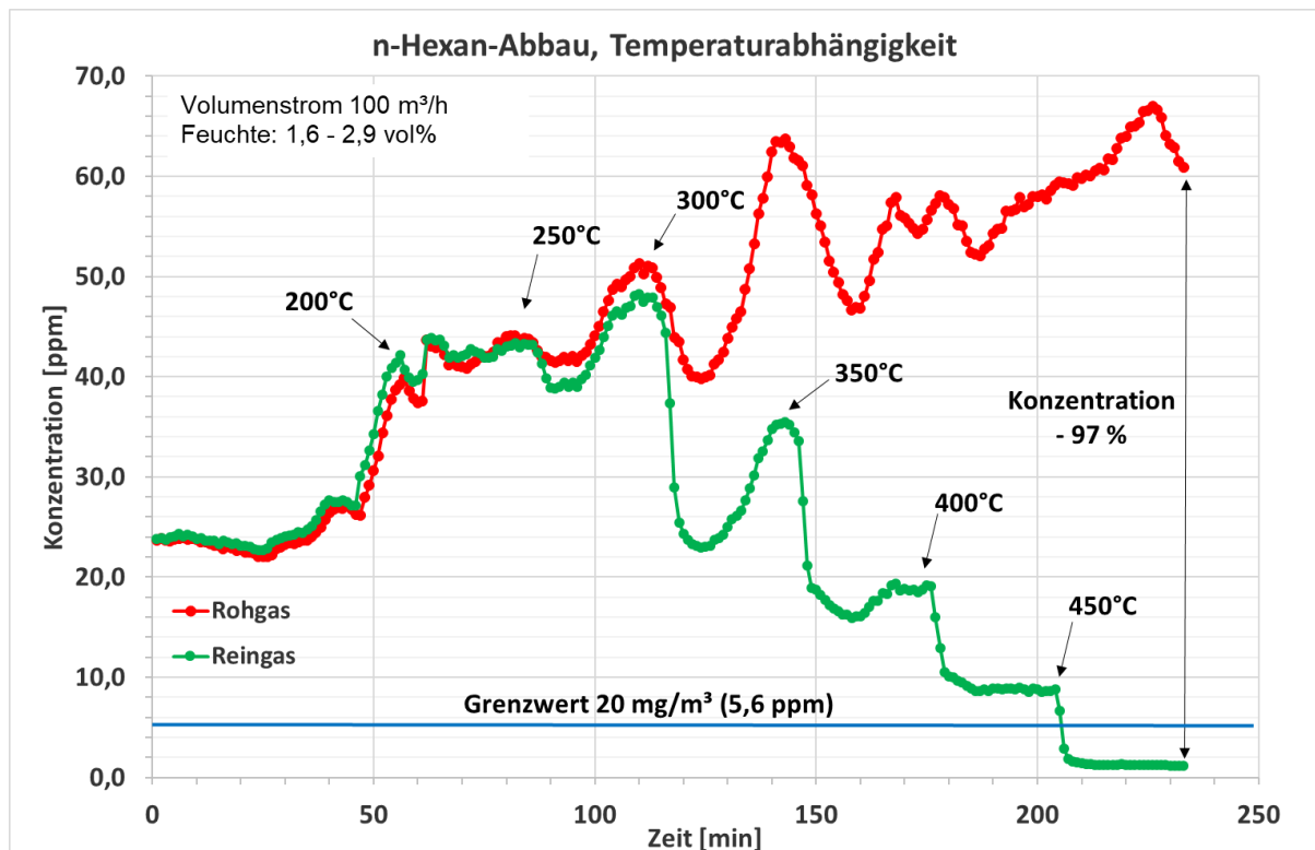
Abbildung 18: Realgasmessung, 100 m³/h Volumenstrom, Variation der Temperatur
