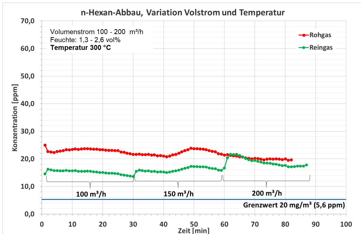
Abbildung 19: Realgasmessung, Temperatur 300°C, Volumenstrom 100, 150, 200 m³/h
