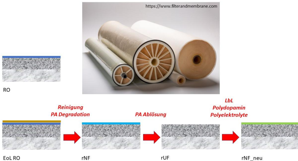
Abb. 1: Schematische Darstellung der unterschiedlichen Arten von Konditionierungsmethoden von EoL-RO-Membranmodulen mit einer Polyamid-Dünnschichtkompositmembran (grau - poröse Trägermembran aus Polysulfon auf Stützvlies; blau - PA-Trennschicht; braun - irreversible Ablagerung / Fouling; hellblau - teilweise degradierte PA-Trennschicht; grün - neu aufgebrachte NF-Trennschicht)
